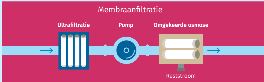
Figuur 3: Schematische weergave van het proces van membraanfiltratie.
