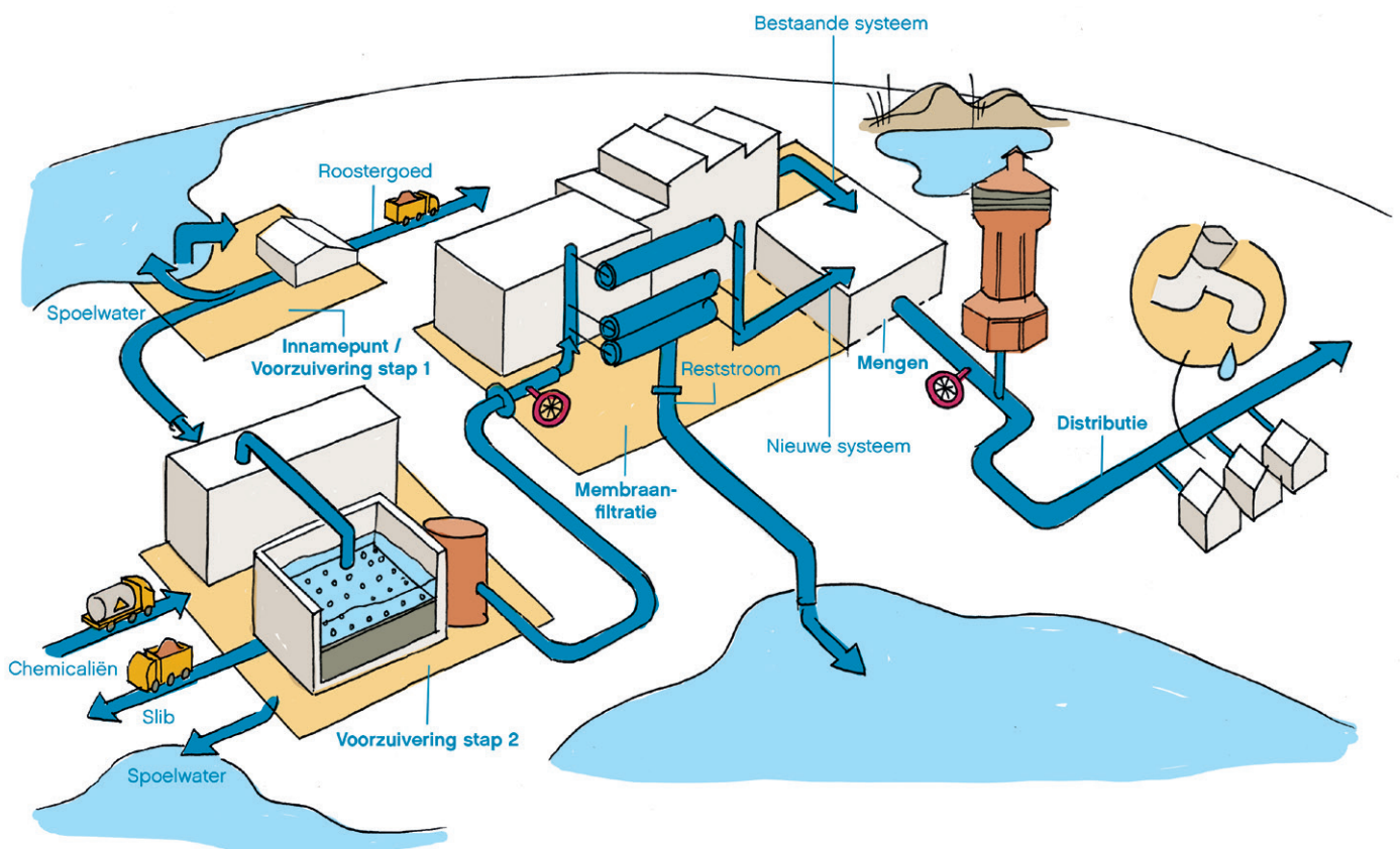
Figuur 7 geeft een ruimtelijk beeld van het hele systeem van inname van water tot en met de distributie van het drinkwater naar de klanten.
